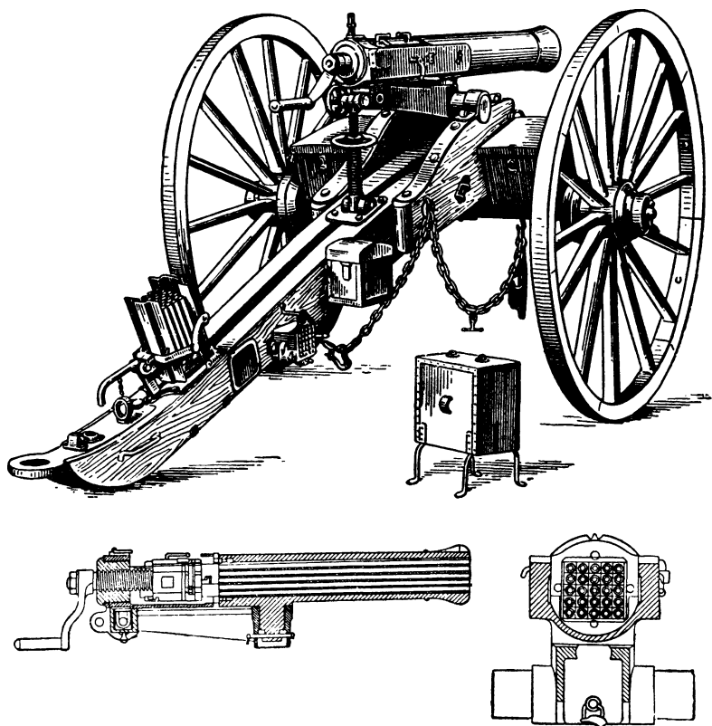
Французская картечица Реффи (рисунки внизу показывают укладку 25 стволов в пять рядов)
