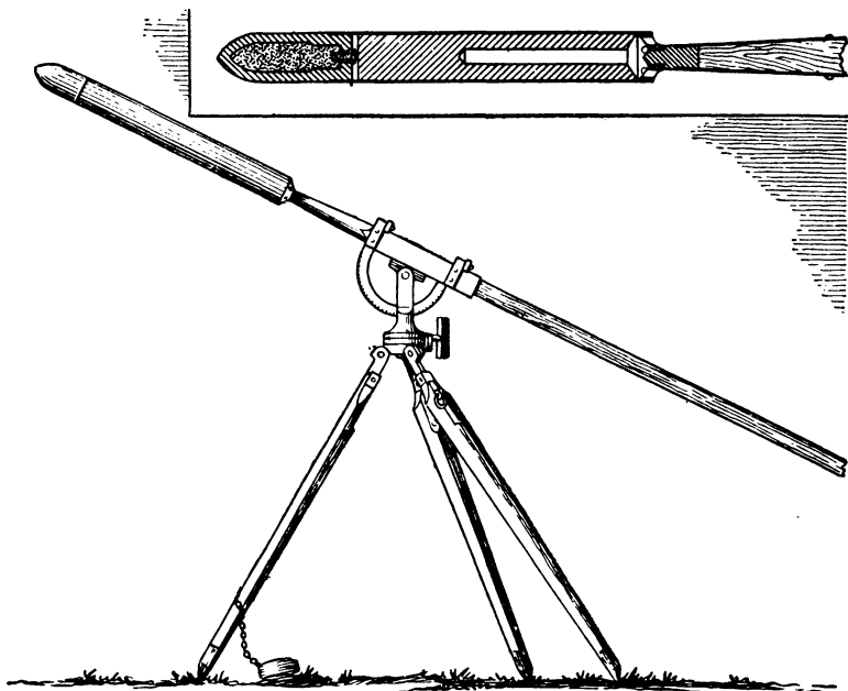
Боевая 2-дюймовая ракета и ракетный станок конструкции К. И. Константинова
