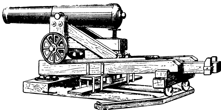
Крепостное орудие на высоком лафете образца 1839 г., на поворотной платформе
